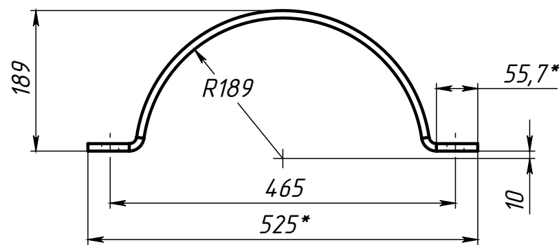
Поз.4 (Полухомут)
